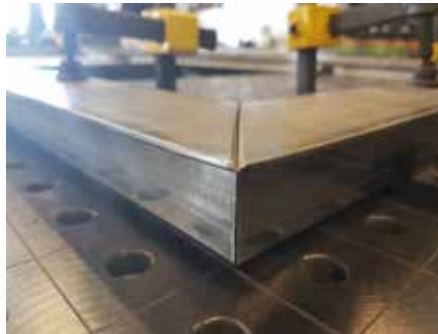
Chanfreinage et assemblage sur les tables de soudure
